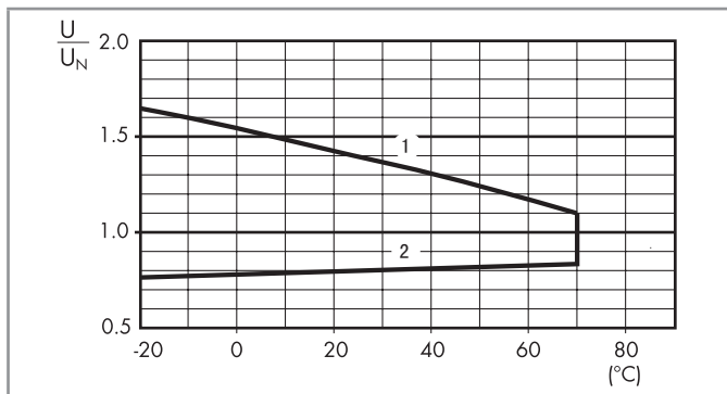
R 58 - AC線圈操作範圍與環境溫度
