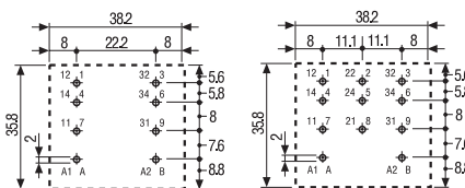
62. 22 PCB銅箔側視圖
