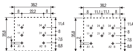
62. 22 - 0300 PCB銅箔側視圖
