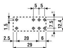
PCB銅箔側視圖
