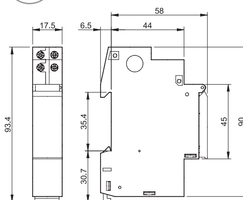
12. 51/12. 81 螺絲終端
